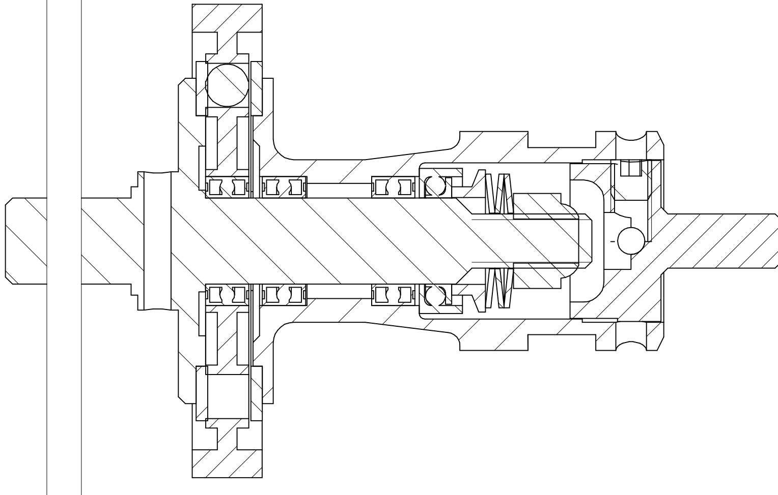
SEZIONE A-A
